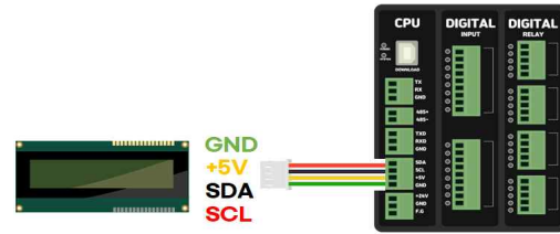
< 캐릭터 LCD 연결 >
